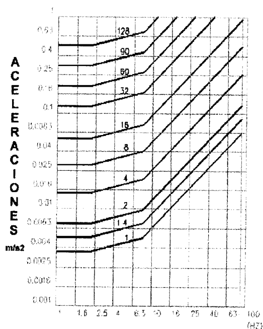
GRÁFICO NÚM. 1 CURVAS BASES DE NIVELES DE INMISIÓN DE VIBRACIONES
