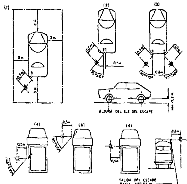
Posiciones para el ensayo de los vehículos parados
